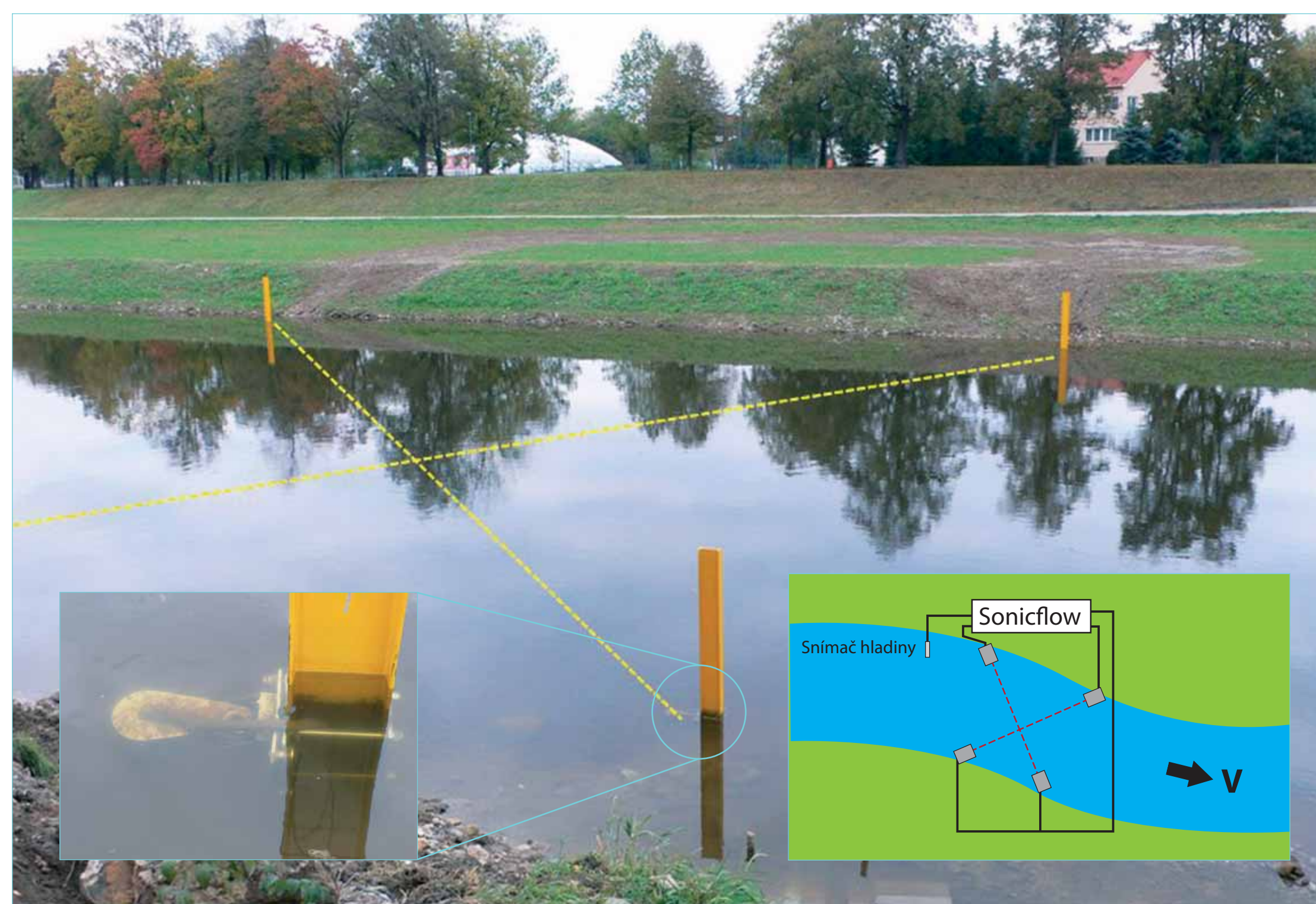
Prohloubení koryta Vltavy v Českých Budějovicích v roce 2009 a regulace hladiny pro umožnění plavby vyřadily z provozu vodoměrnou stanici. Právě tady byl instalován první stabilní ultrazvukový průtokoměr. Pro vyšší spolehlivost a přesnost měření využívá čtveřici snímačů a dvojici zkřížených ultrazvukových paprsků.
